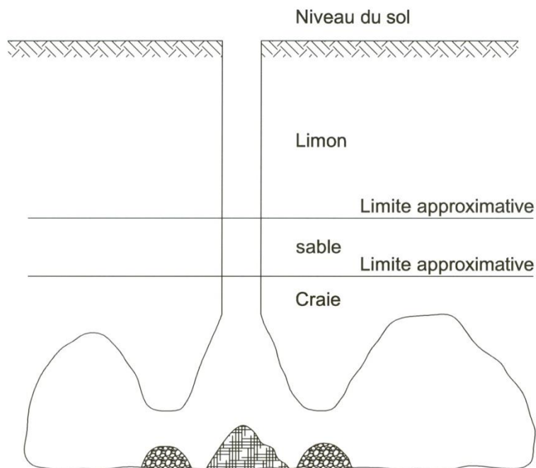
Coupe AA'
